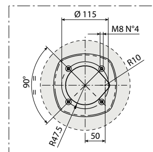
Vista parziale da C Partial view from C
