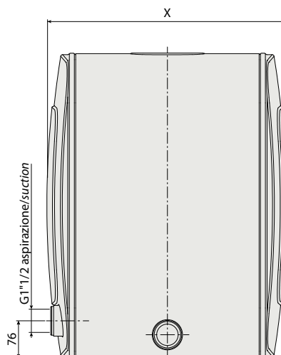
Vista parziale da C Partial view from C
